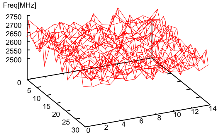
チップ内ばらつき特性( \sigma/\mu=1.6\% )
